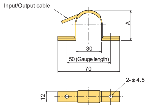
PI-2-50/PI-5-50
