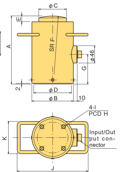
CLP-1~ 5MNB
