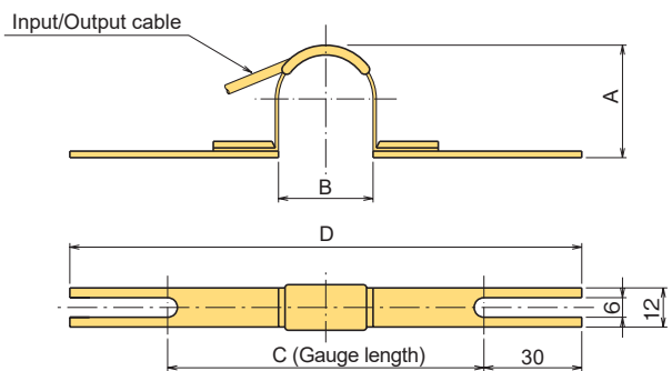
PI-2/PI-5
