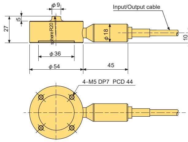
CLR-50~ 200KNAH
